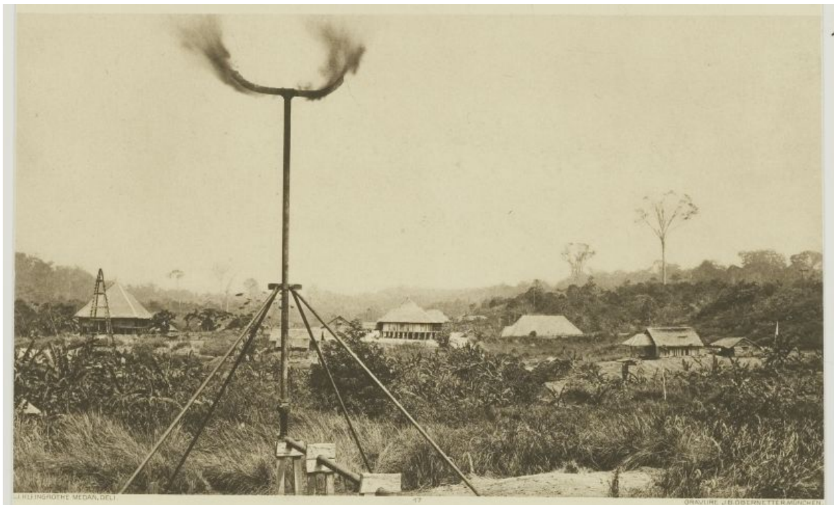
Verbranding van aardgas op een olieboorlocatie, vermoedelijk in Pangkalan Brandan, oostkust van Sumatra.
